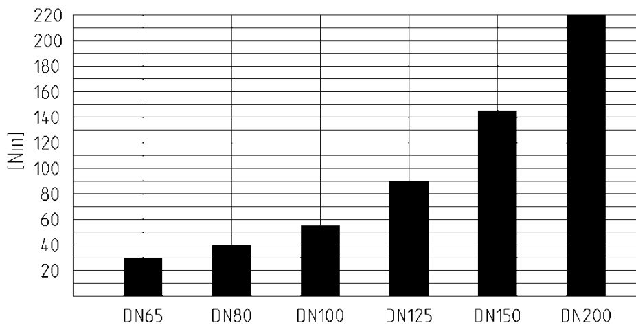
Anzugsdrehmoment der
